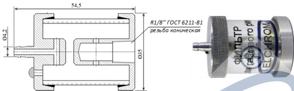
Рисунок 12. Фильтр (маслоуловитель)
